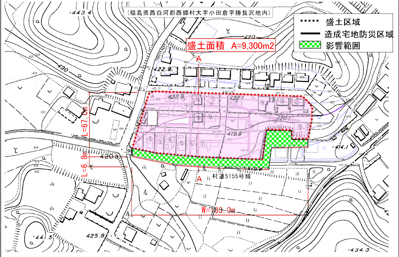
平面図（造成宅地滑動崩落緊急対策工事） S=1:2,500程度
